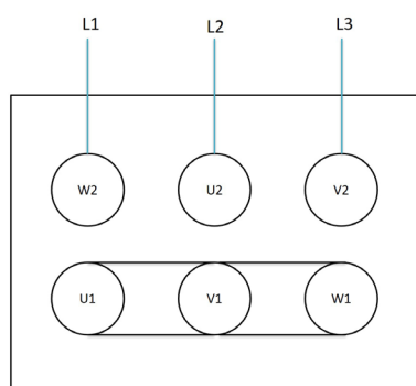
Mała liczba biegunów- połączenie Dahlandera (YY)
