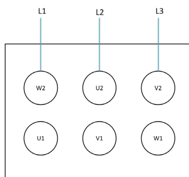
Mała liczba biegunów- połączenie rozdzielne (Y/Y)
