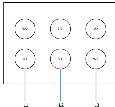
Duża liczba biegunów - połączenie w gwiazdę (Y)
